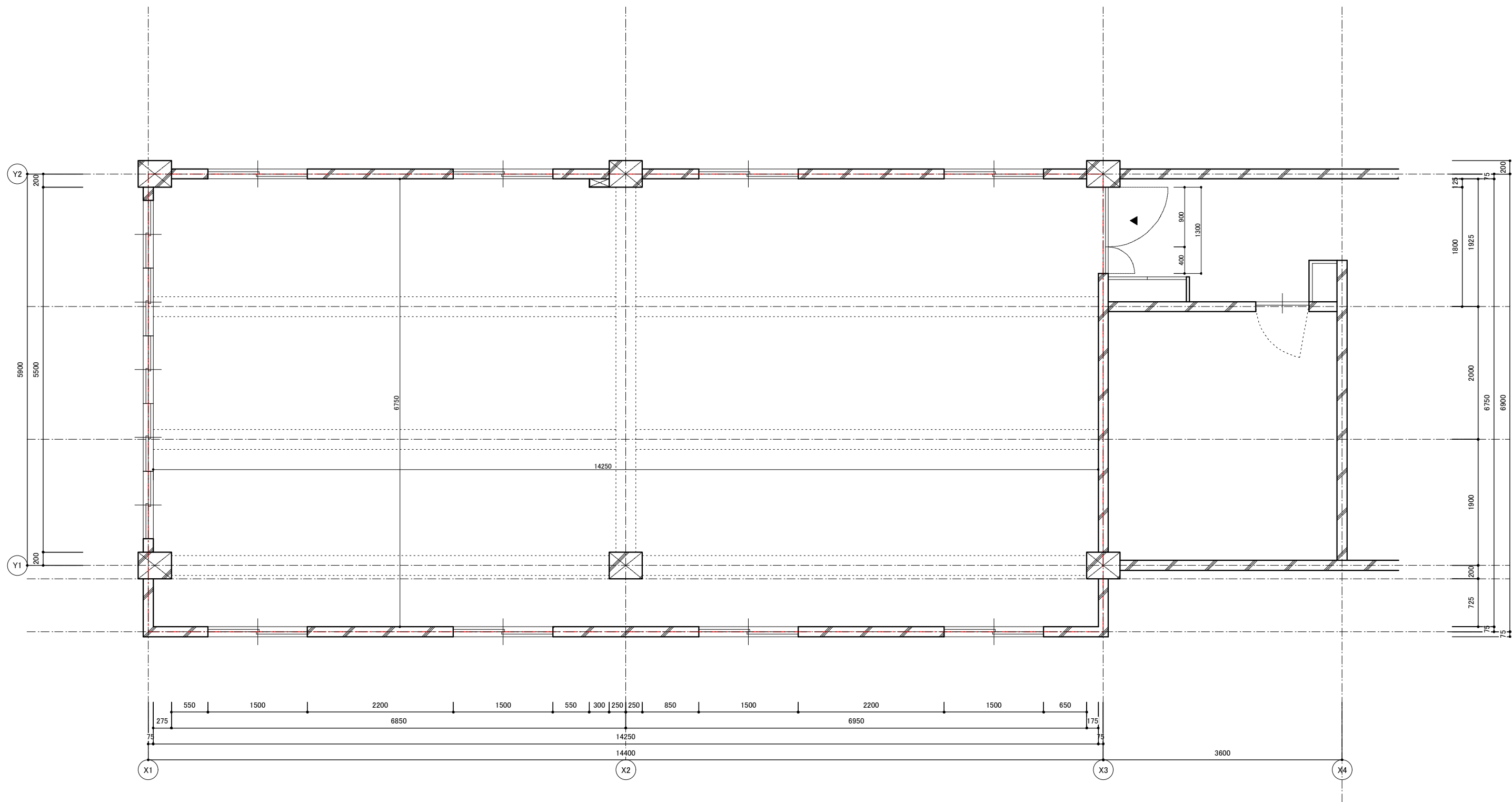
平面图 Scale=1/60
